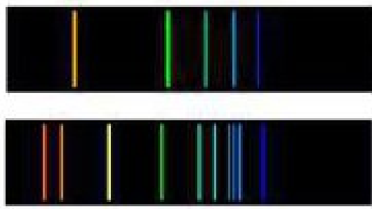
Abbildung 1: Emissionslinien von Wasserstoff (oben) und Helium (unten)
